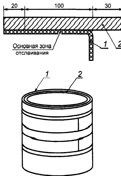
1 - защитное покрытие; 2 - металлическая подложка (труба)
